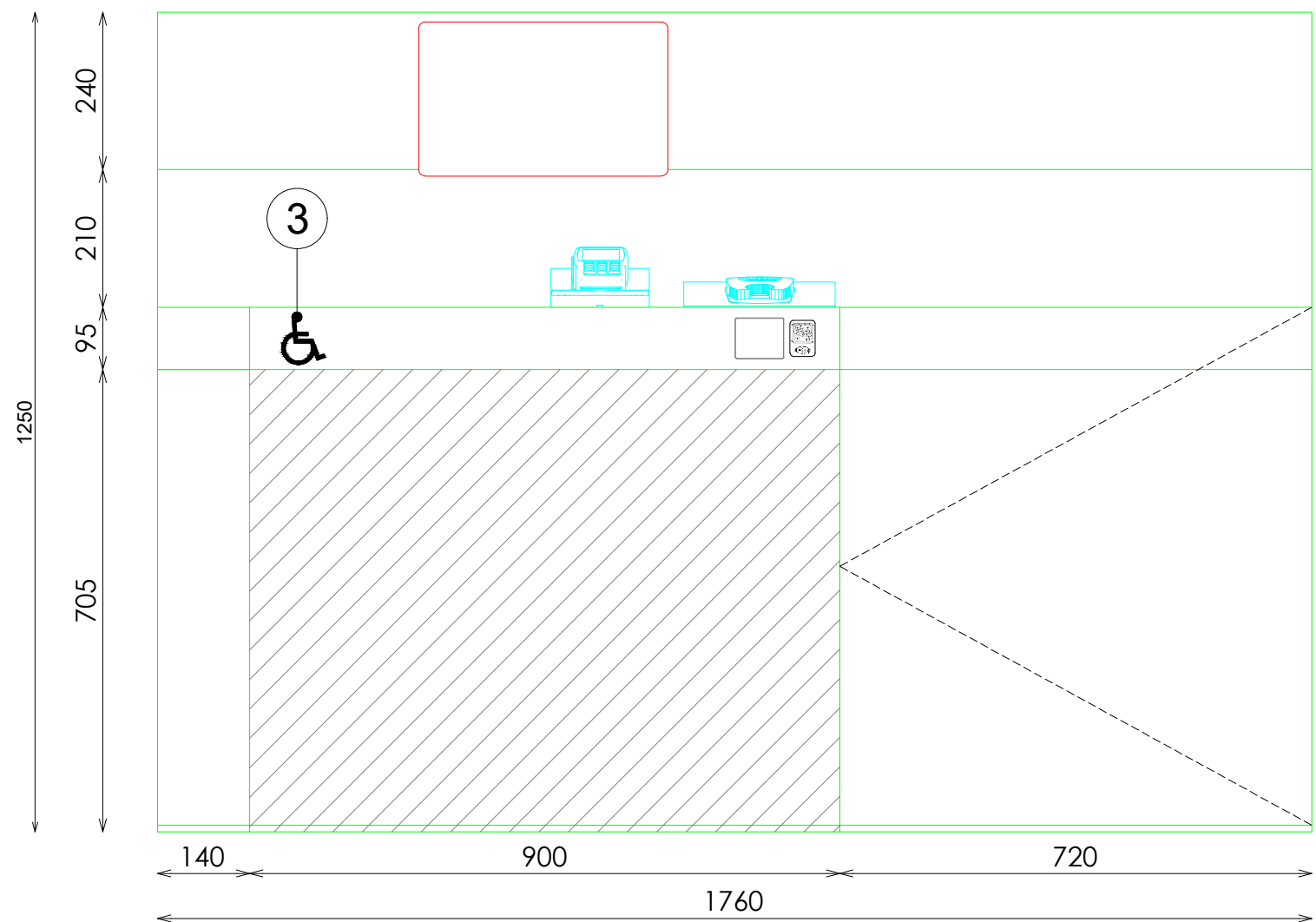
ALZADO
