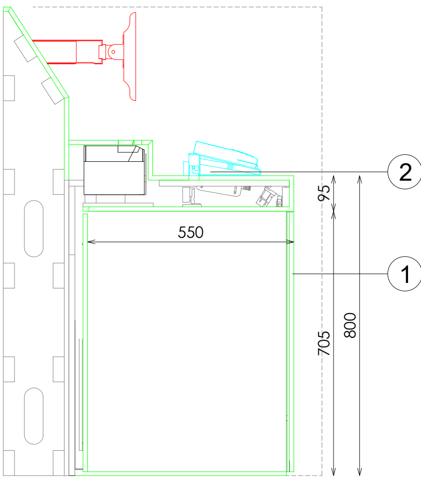
SECCION
