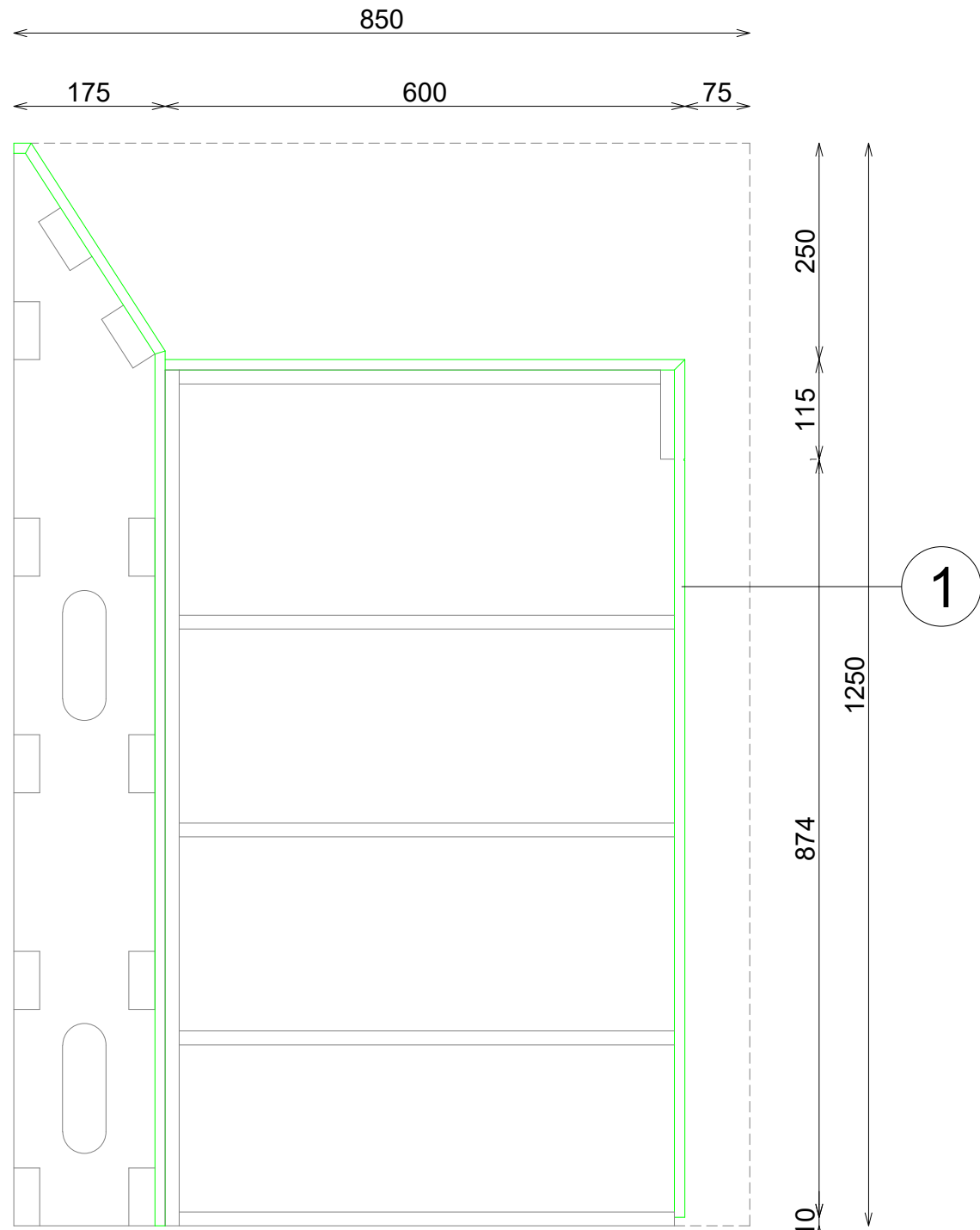
SECCION
