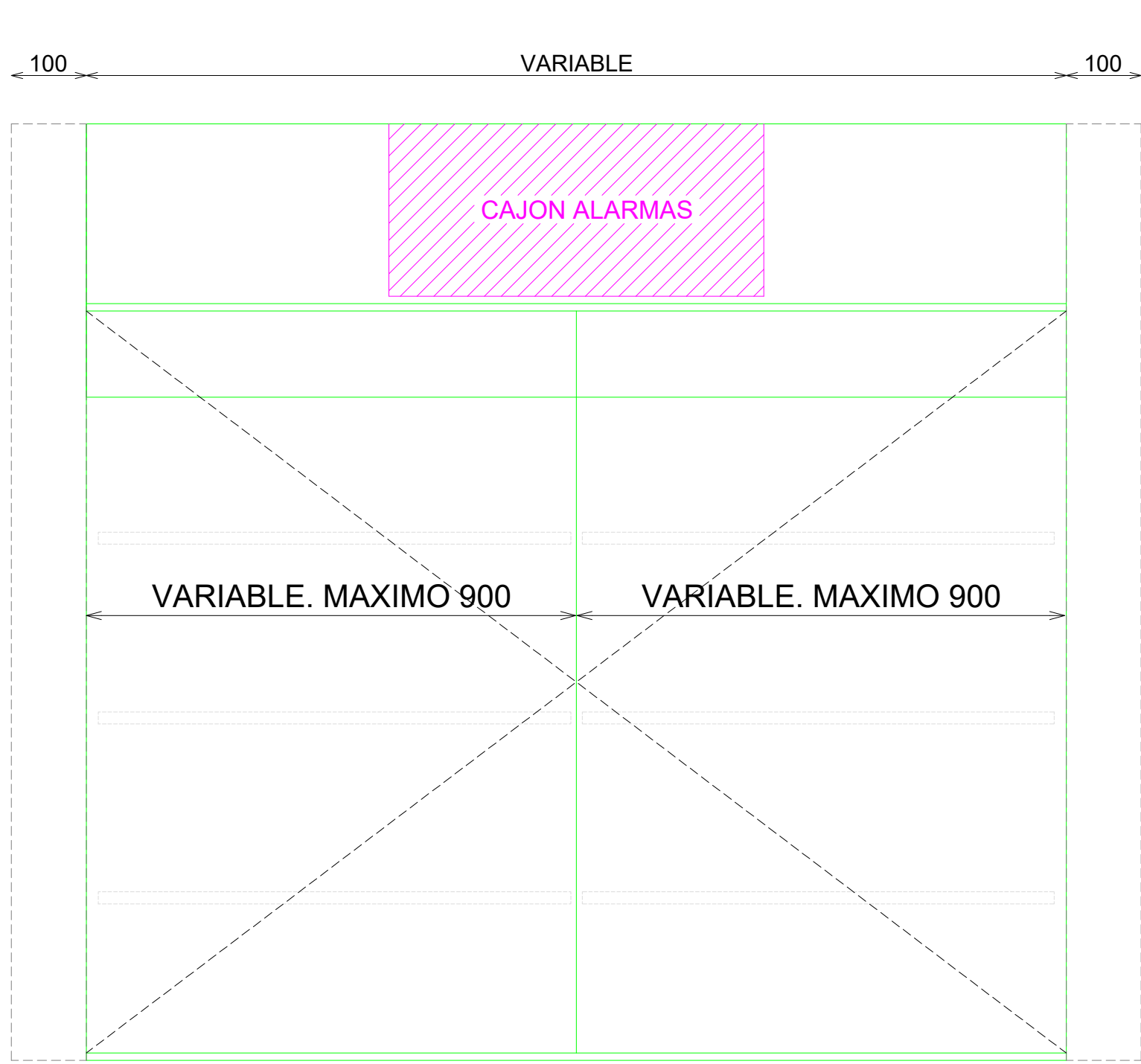
ALZADO FRONTAL
