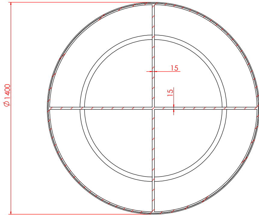
剖面 AH-AH
