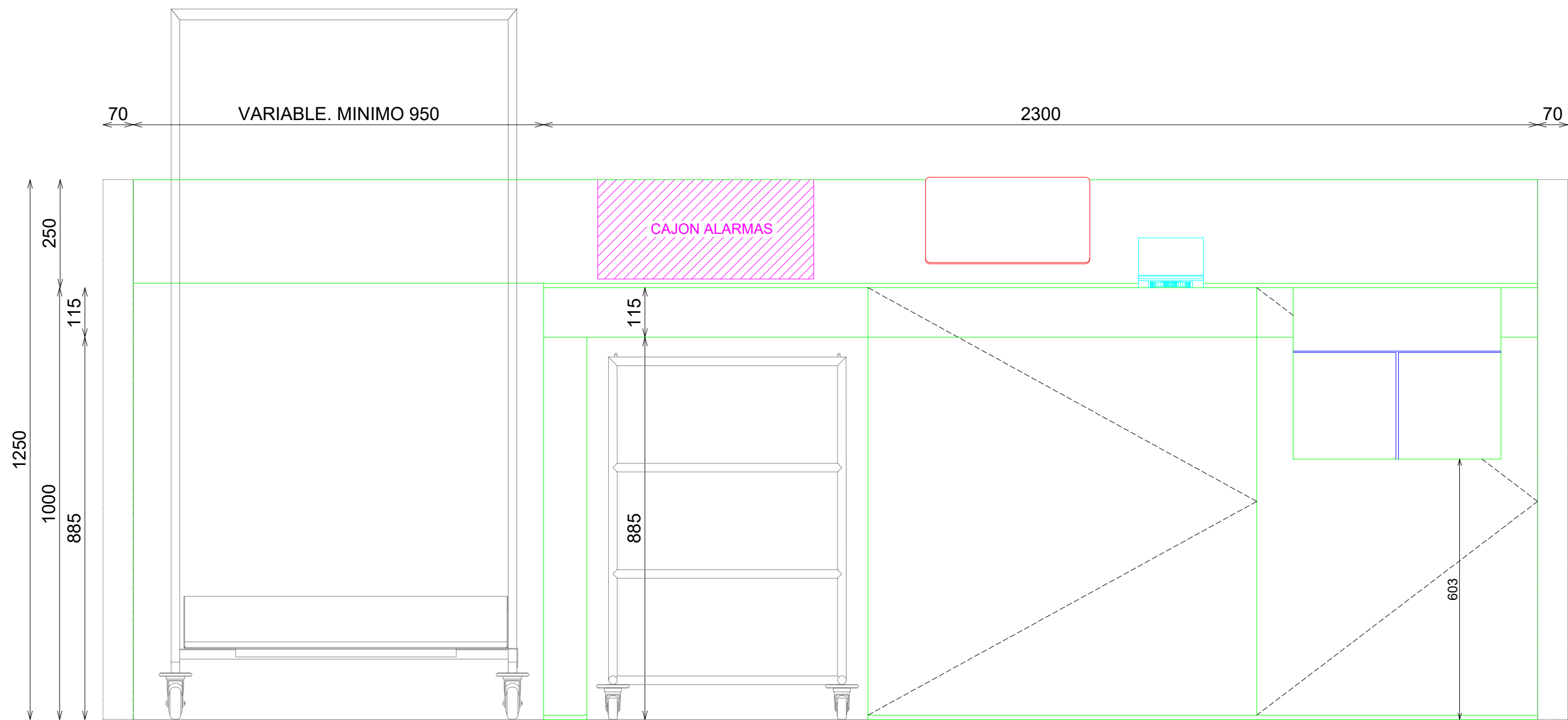
ALZADO FRONTAL
