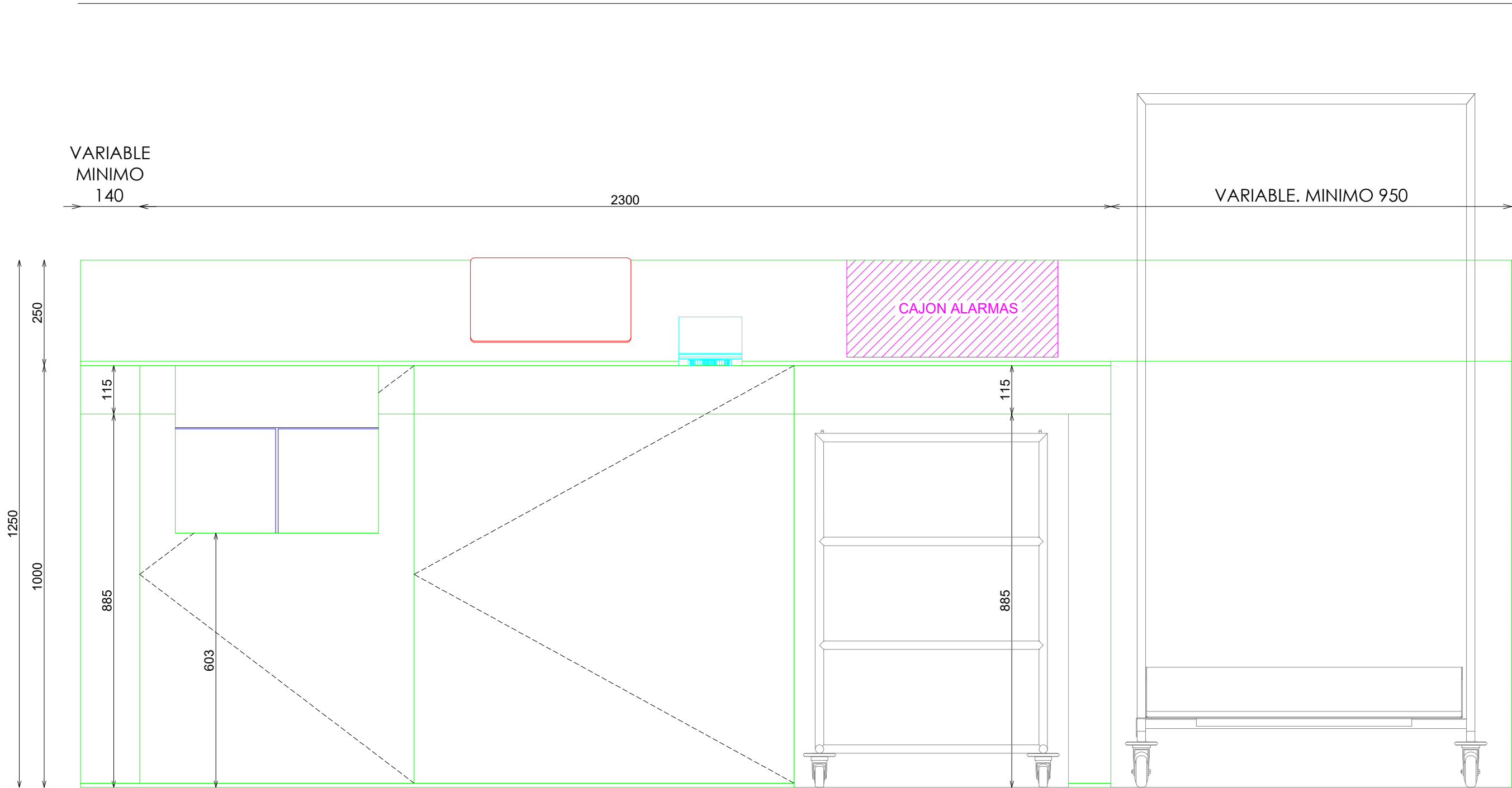
ALZADO FRONTAL
