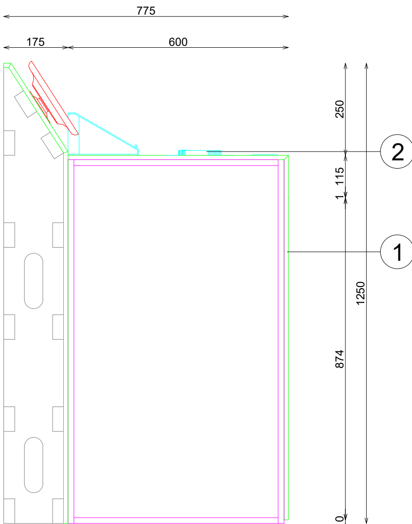
SECCION
