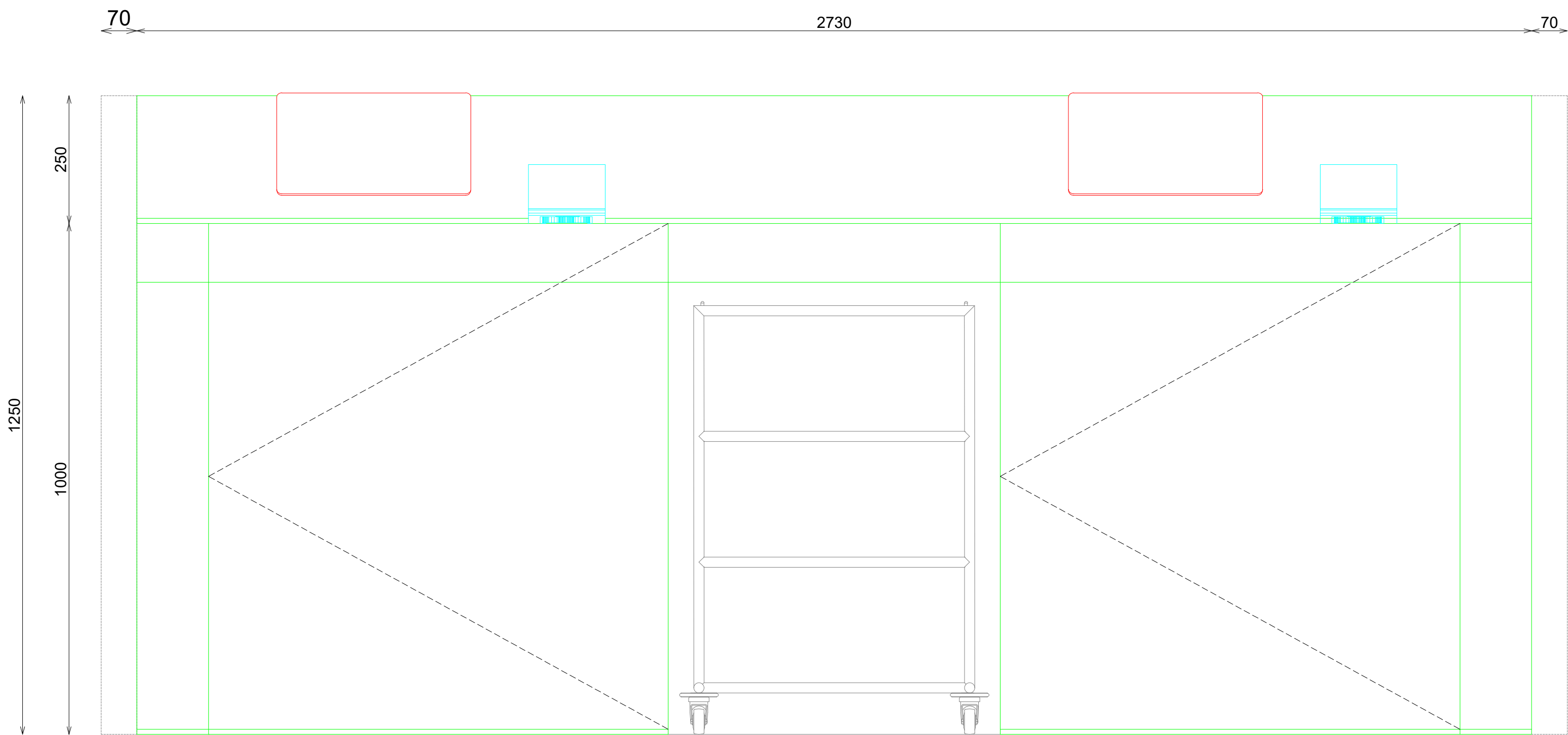
ALZADO FRONTAL
