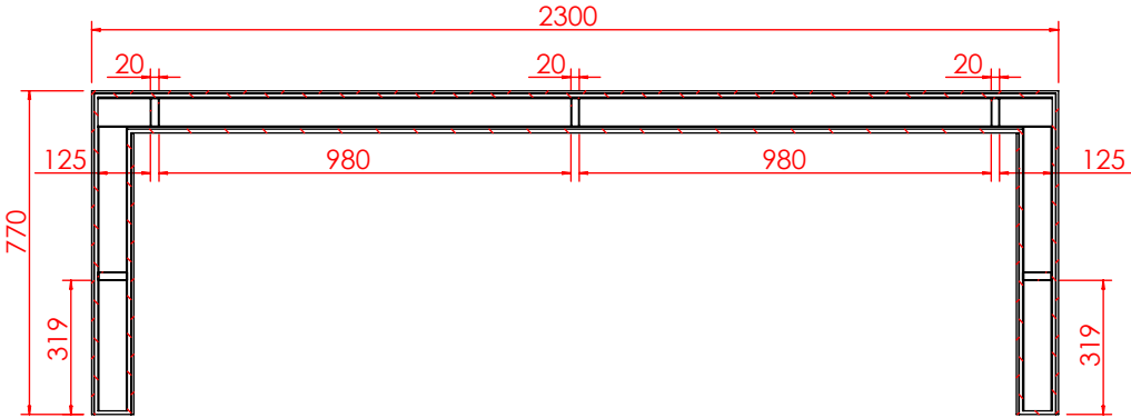
剖面 AG-AG
