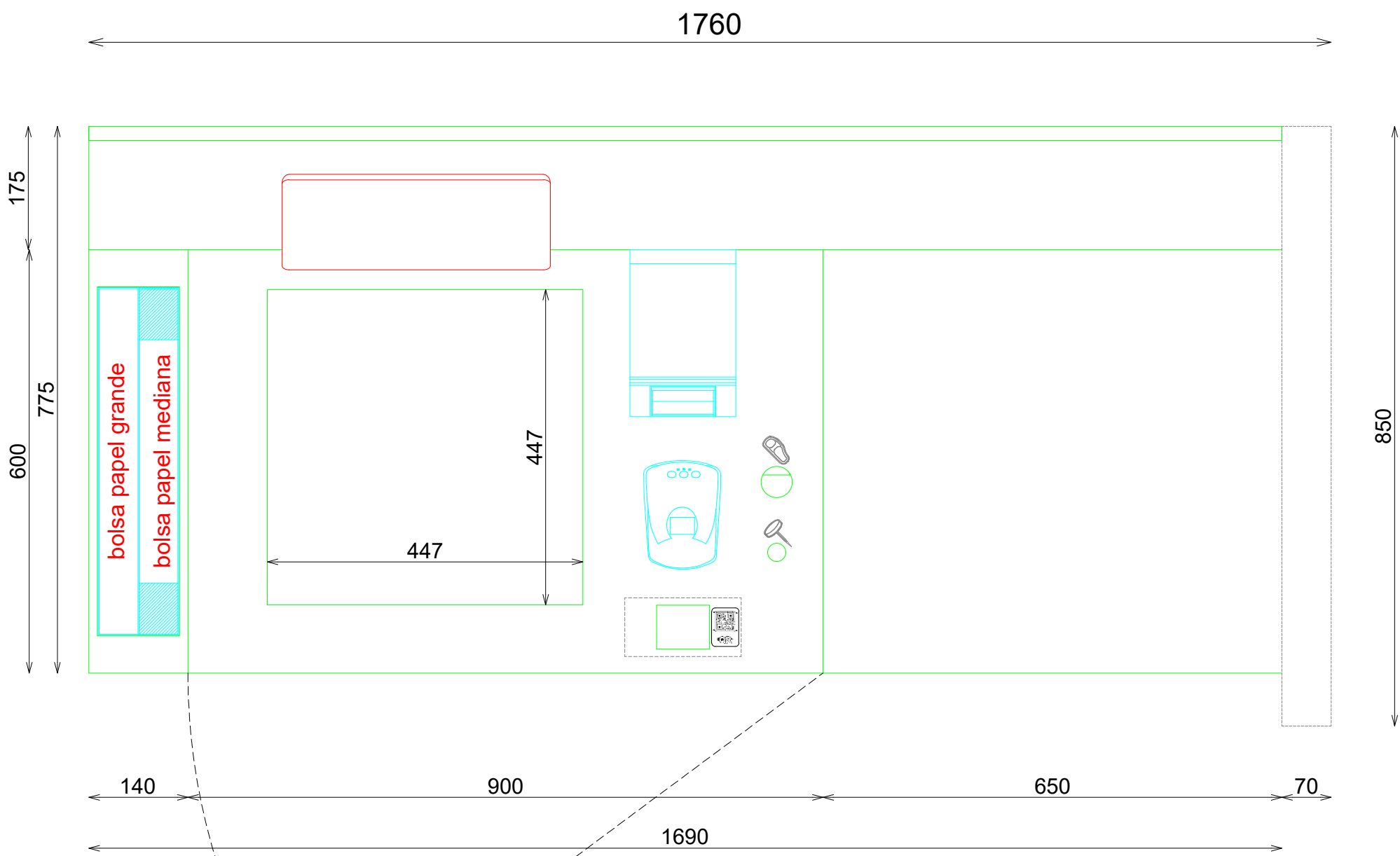
PLANTA
