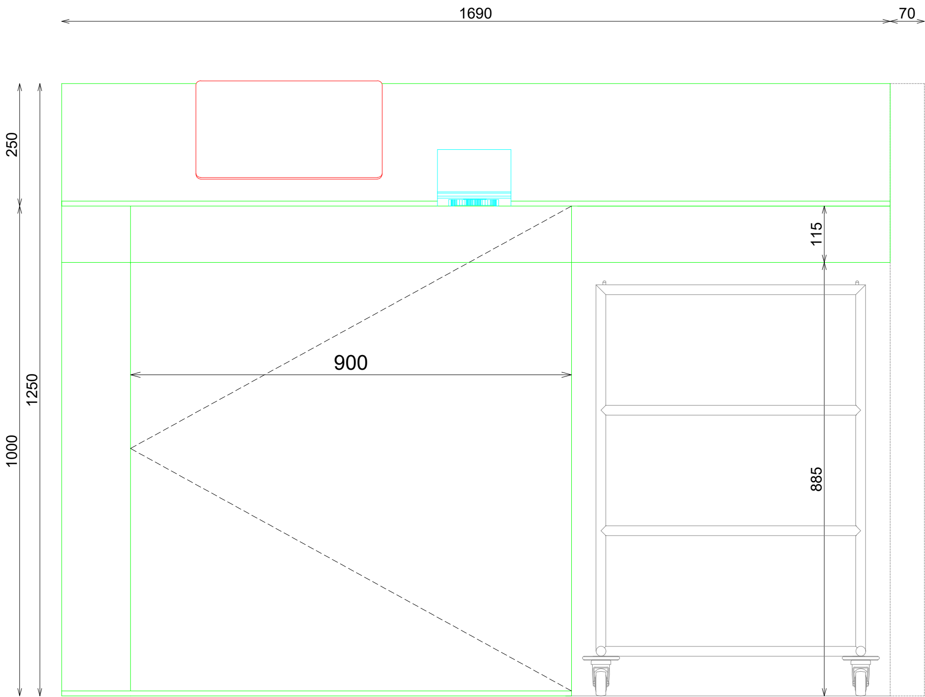
ALZADO FRONTAL
