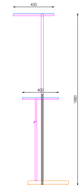
ALZADO LATERAL
