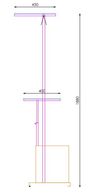
SECCIÓN (ANCLAJE PARED)
