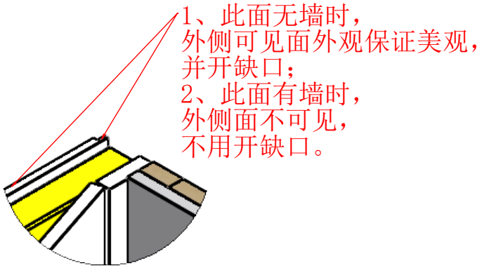
局部视图 AG 比例 1:5
