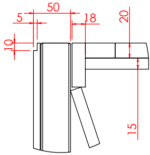
局部视图 AH 比例 1:5
