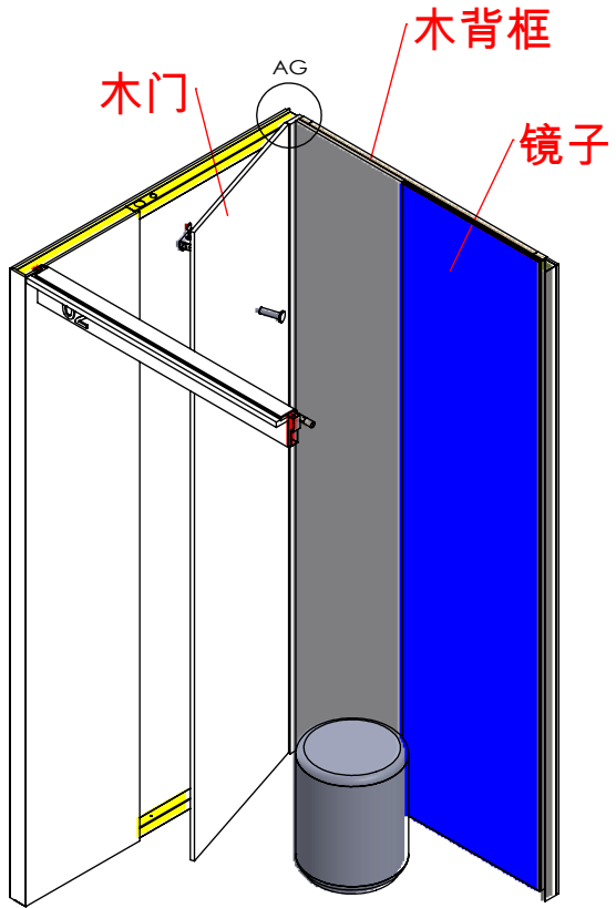
局部视图 AG 比例 1:5
