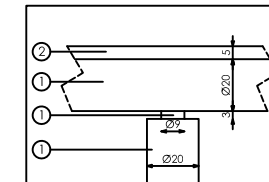
DETALLE B
