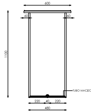
ESTRUCTURA
