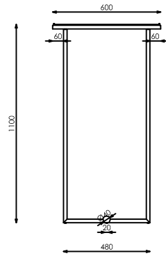
ALZADO
