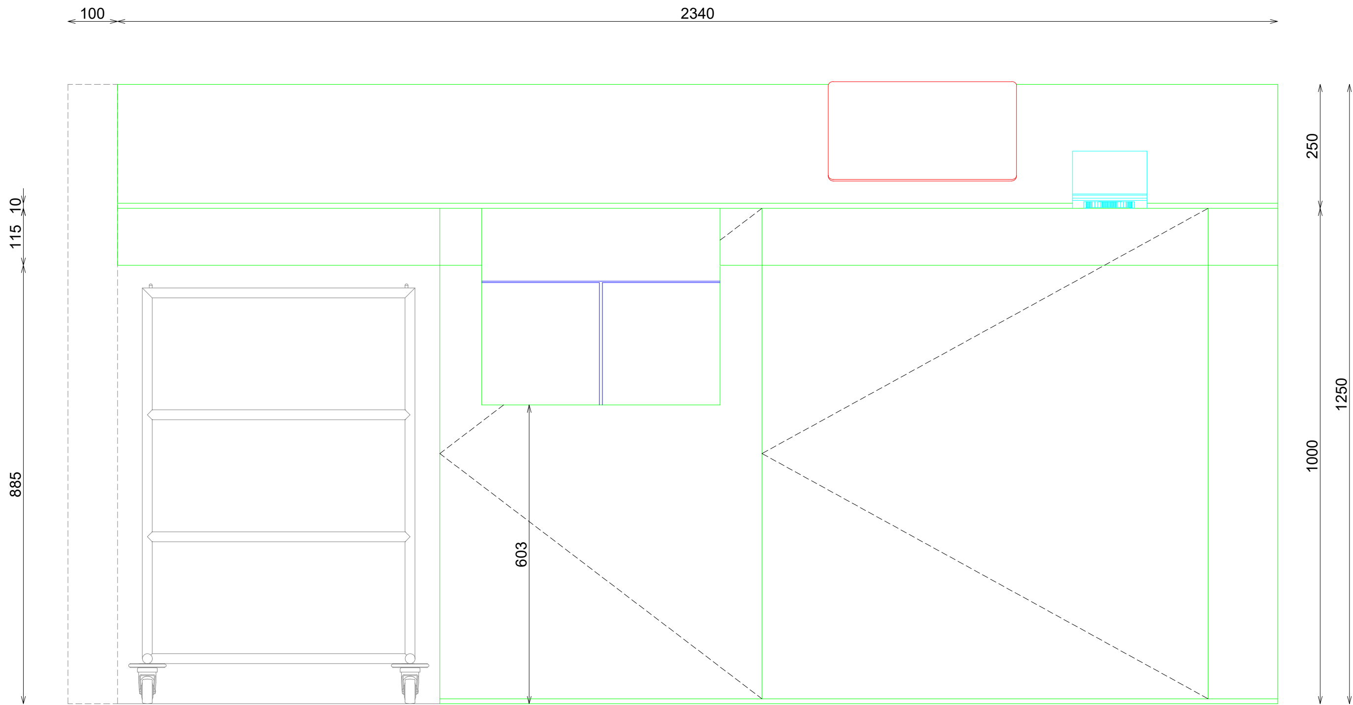
ALZADO FRONTAL
