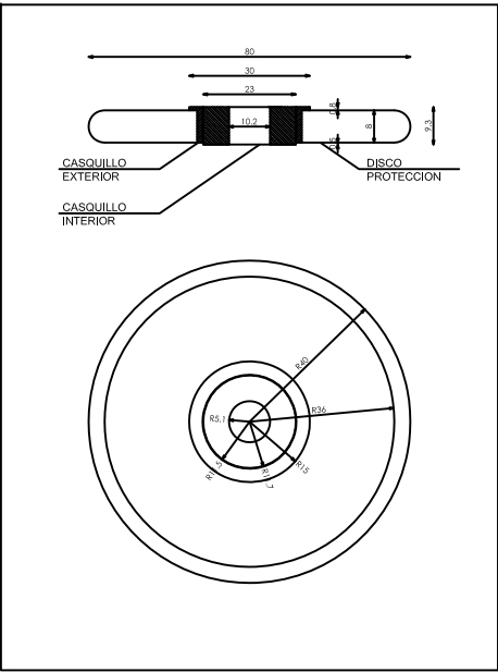
DETALLE DISCO PROTECCION
