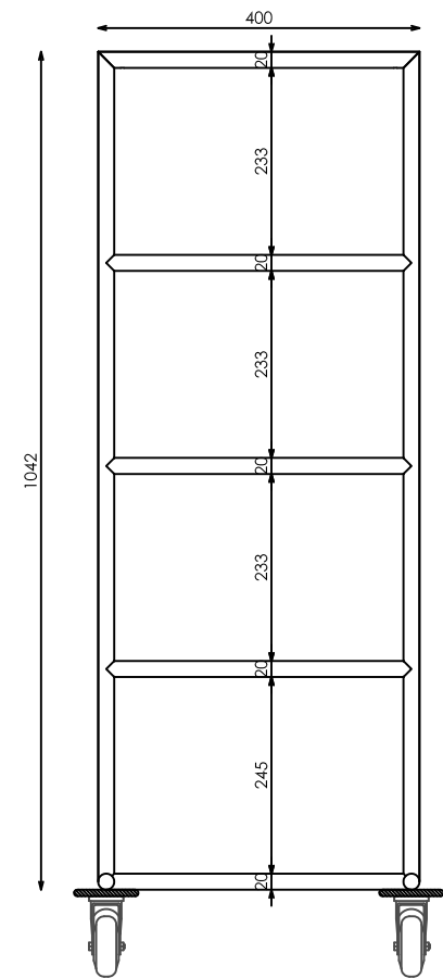
ALZADO FRONTAL
