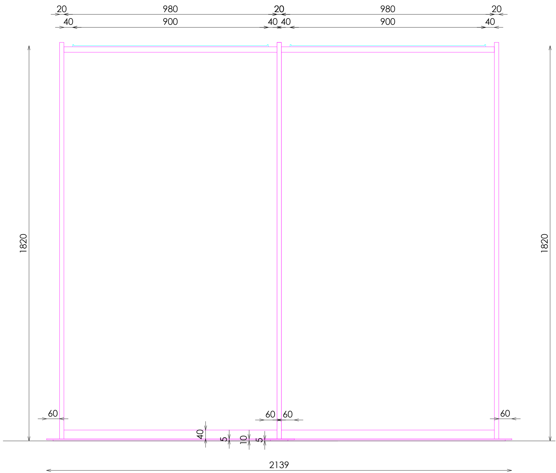
ALZADO
