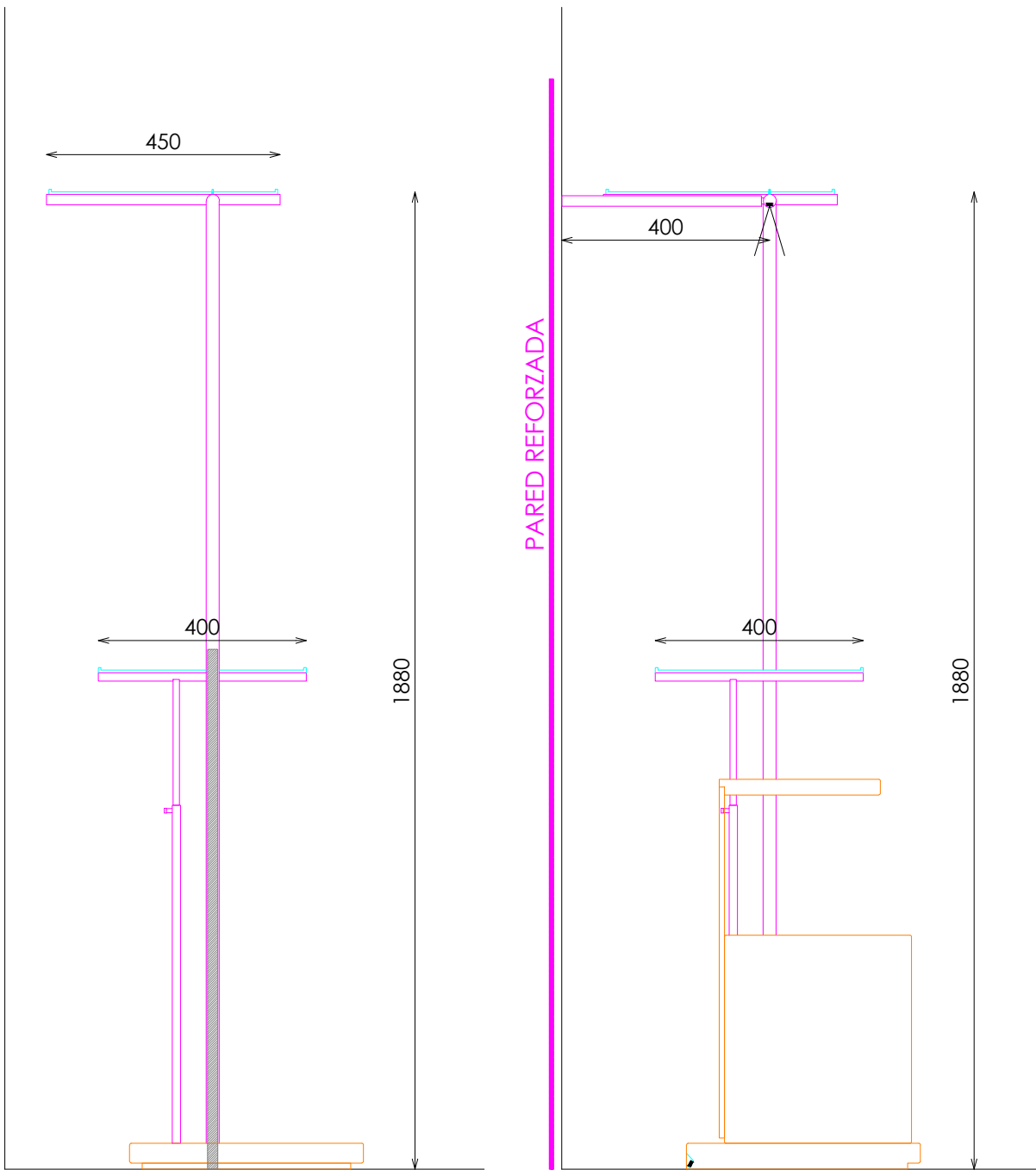
ALZADO LATERAL
