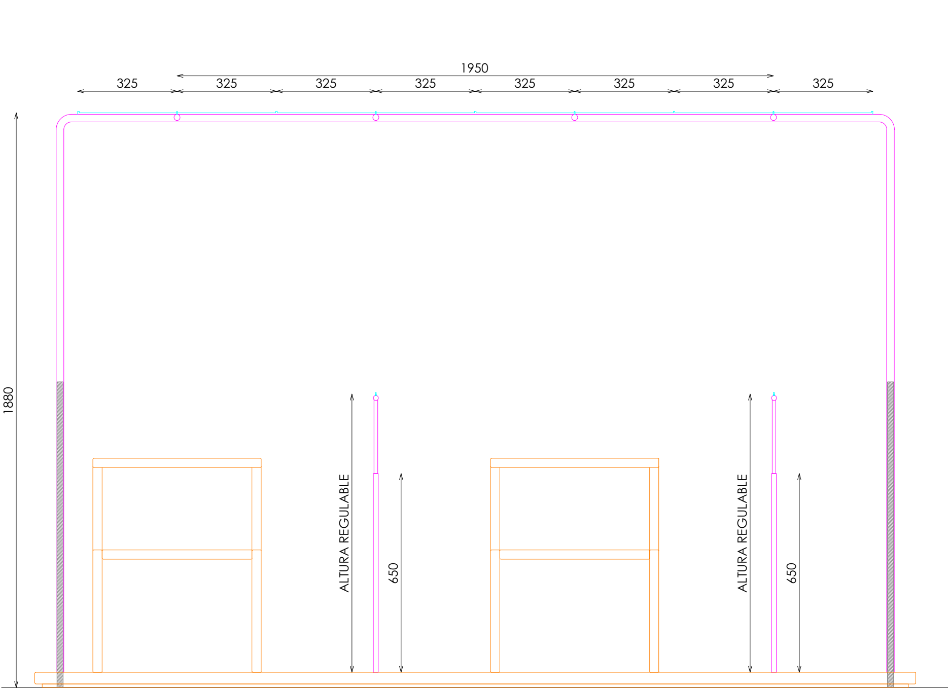
ALZADO FRONTAL
