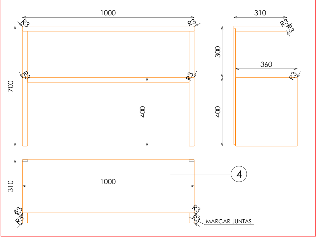
SECCIÓN
