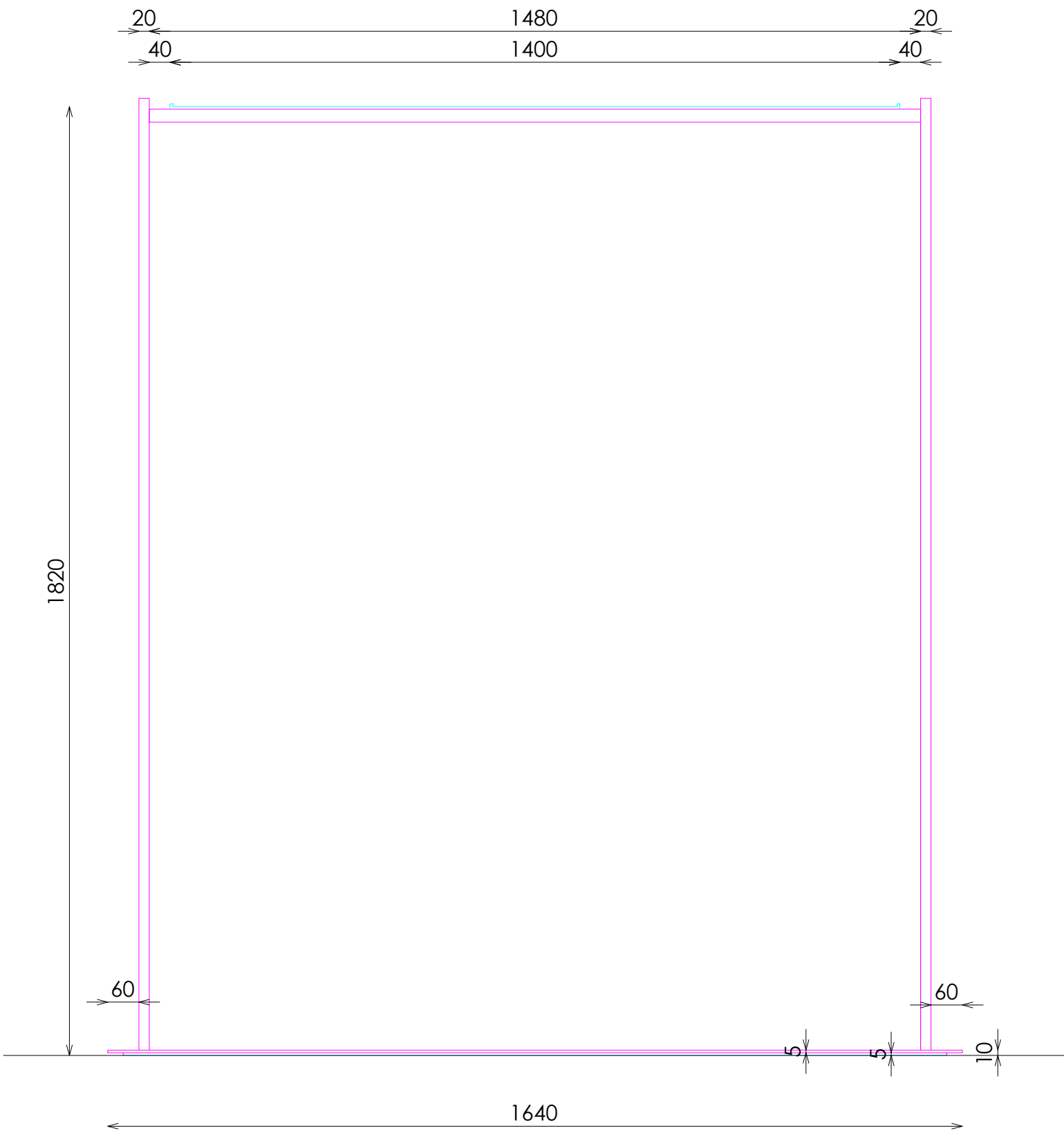
ALZADO
