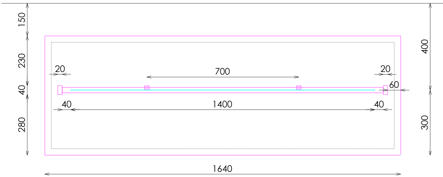
PLANTA
