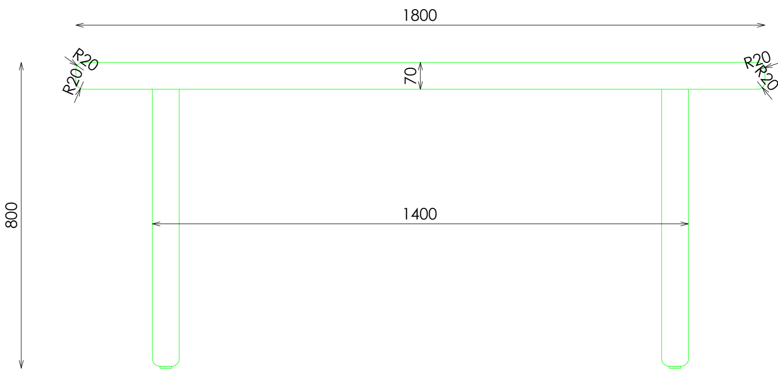
ALZADO
