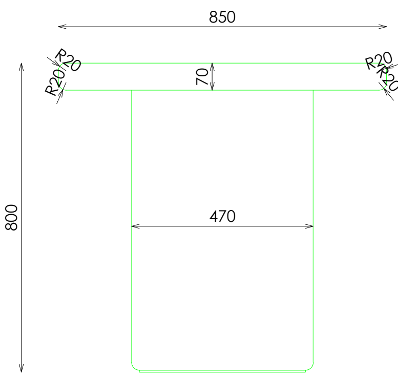
PERFIL
