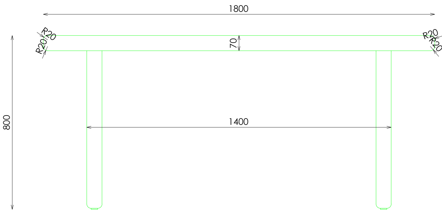
ALZADO
