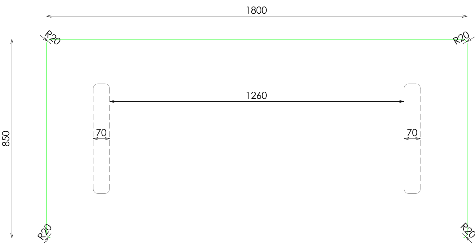
PLANTA
