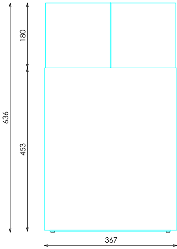
ALZADO
