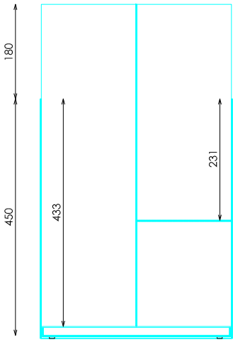
SECCION
