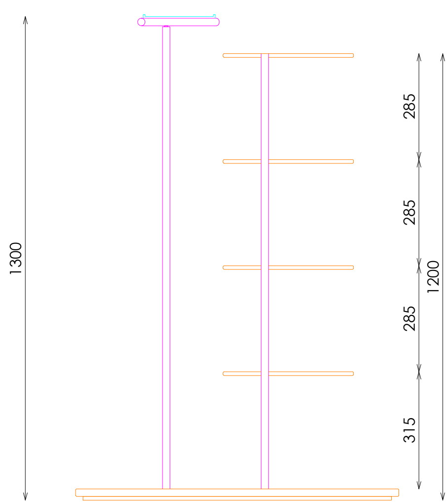
ALZADO
