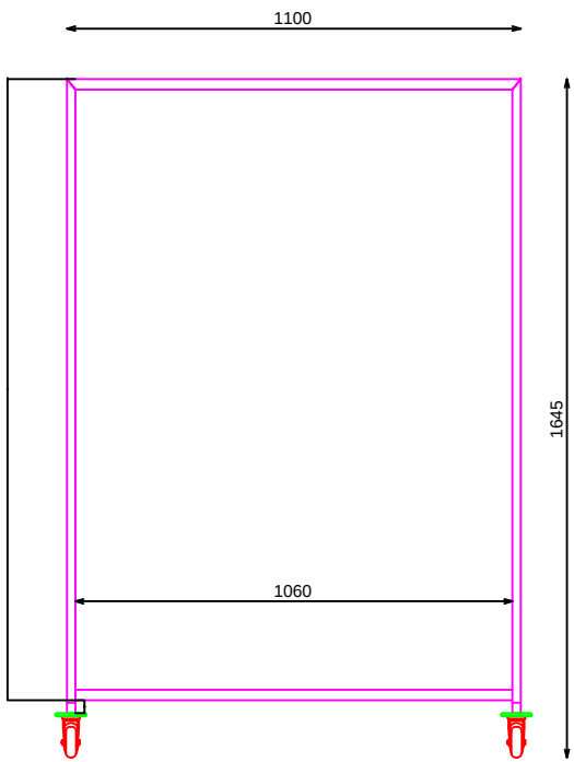
ALZADO FRONTAL
