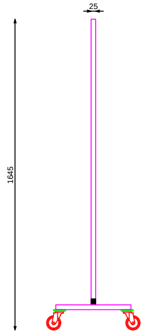
ALZADO LATERAL
