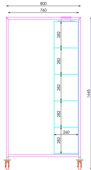
ALZADO FRONTAL
