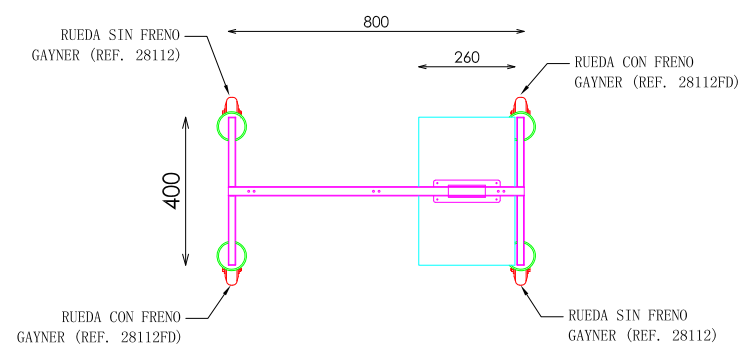
PLANTA
