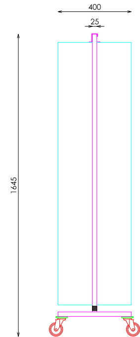
ALZADO LATERAL
