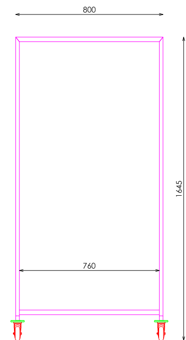
ALZADO FRONTAL
