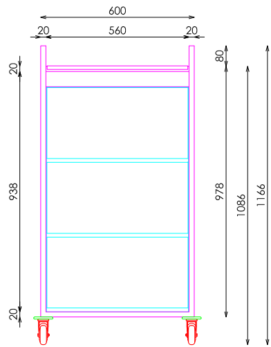
ALZADO FRONTAL
