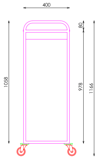
ALZADO LATERAL
