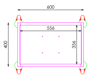
PLANTA BANDEJA
