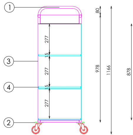
SECCION
