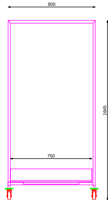
ALZADO FRONTAL
