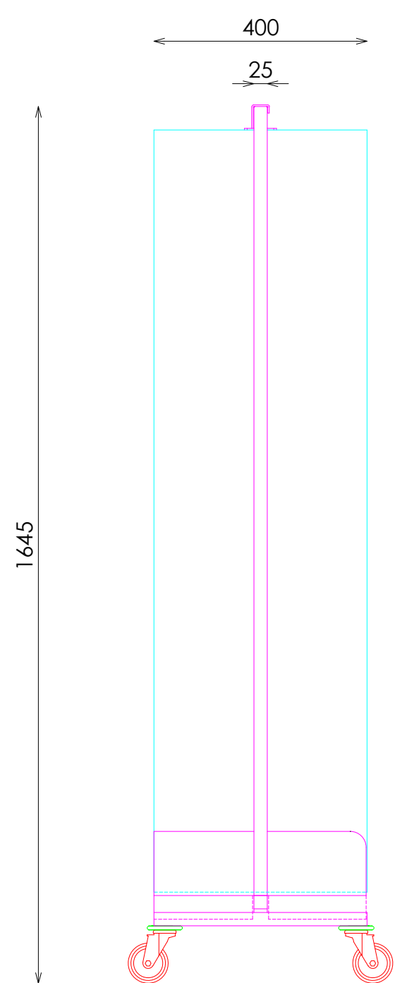
ALZADO LATERAL
