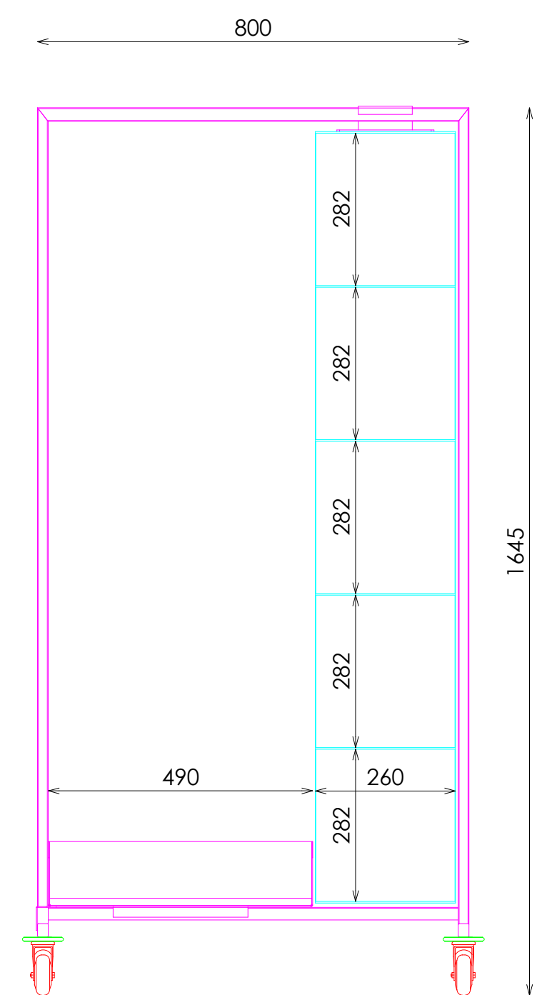
ALZADO FRONTAL
