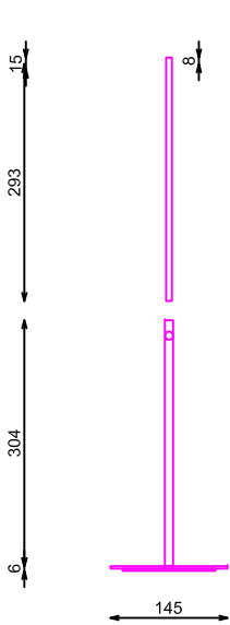
ALZADO C
