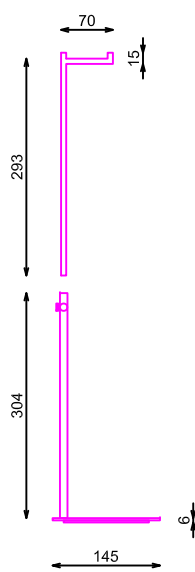
ALZADO D
