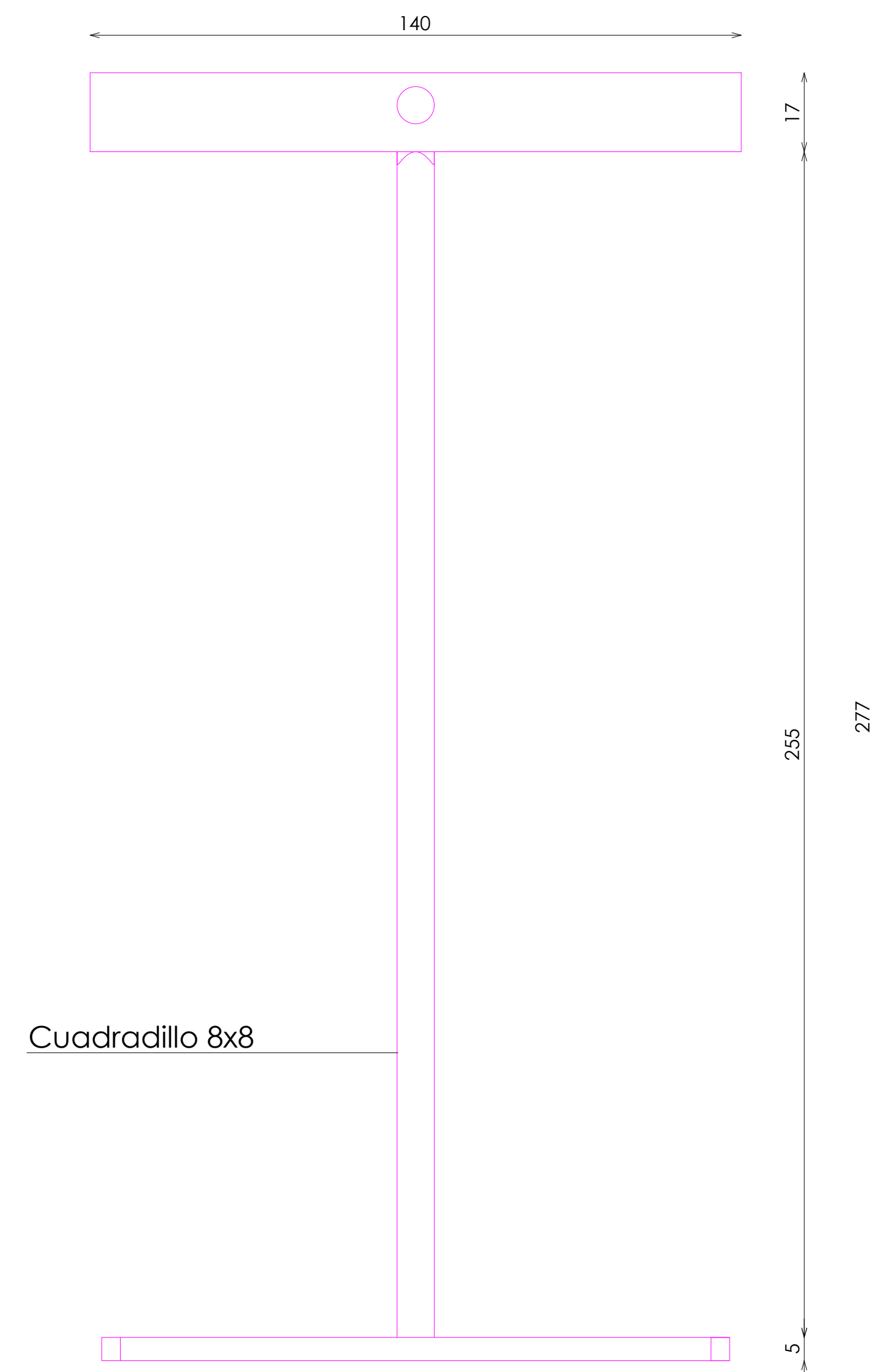
ALZADO
