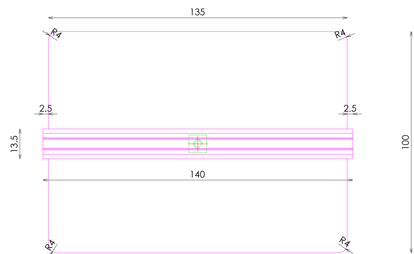
PLANTA
