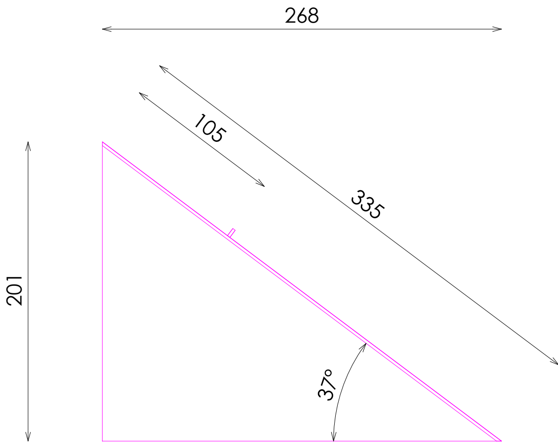
SECCIÓN
