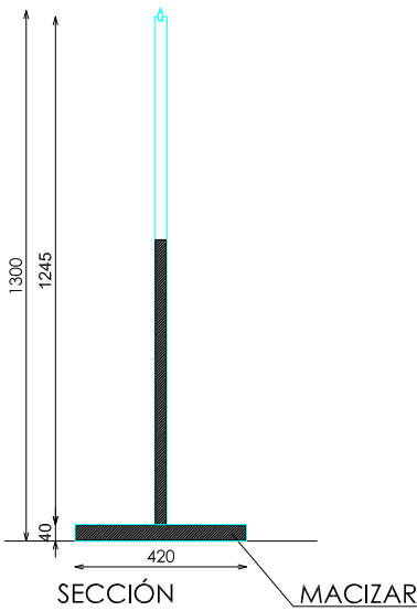
SECCIÓN
