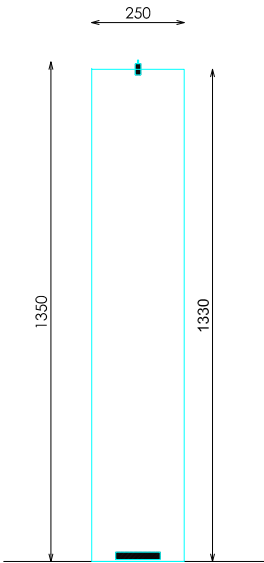
SECCION
