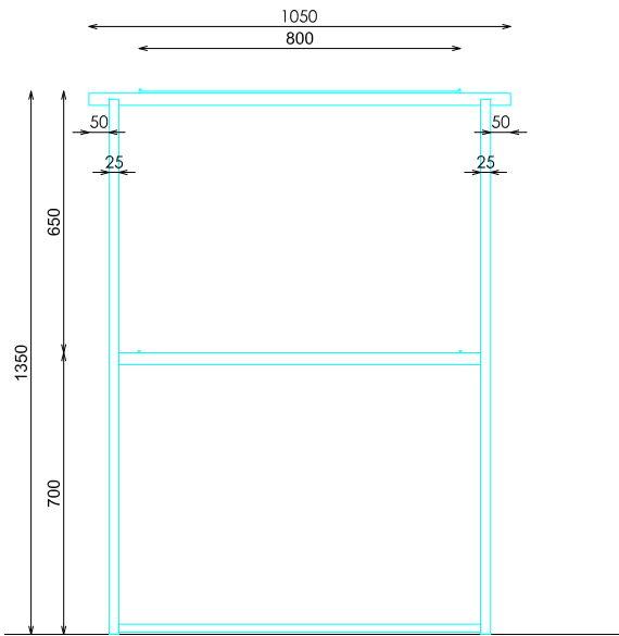
ALZADO
