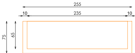
SECCION PERFIL
