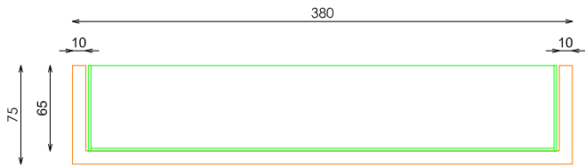
SECCION LONGITUDINAL
