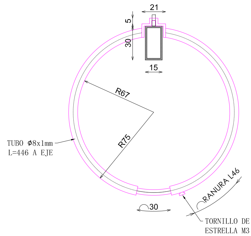
ALZADO
