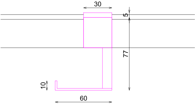
ALZADO
