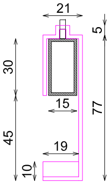
SECCIÓN
