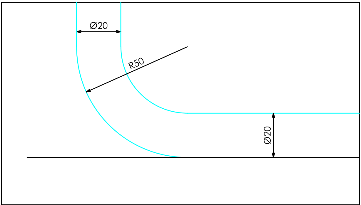
DETALLE D (ESQUINAS INFERIORES)
