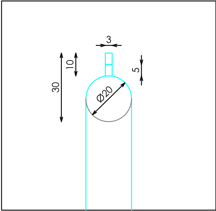
DETALLE A
