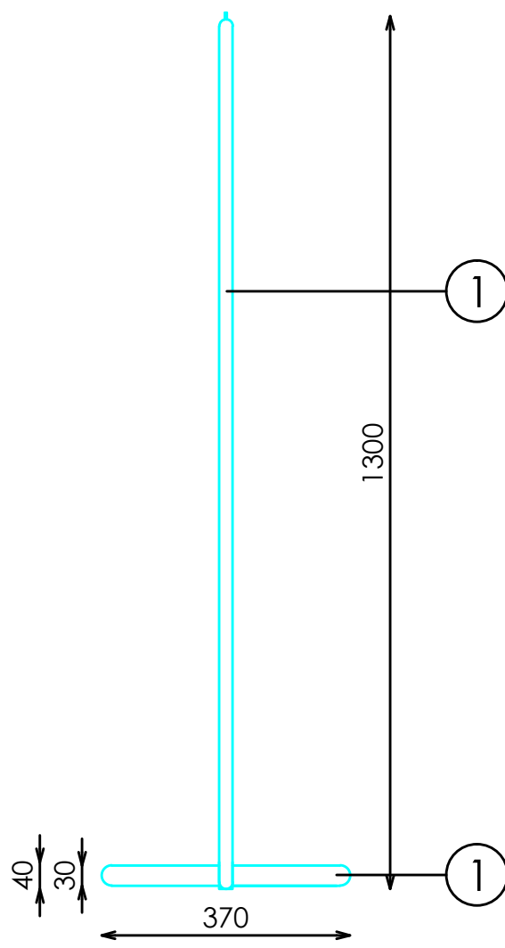
PERFIL
