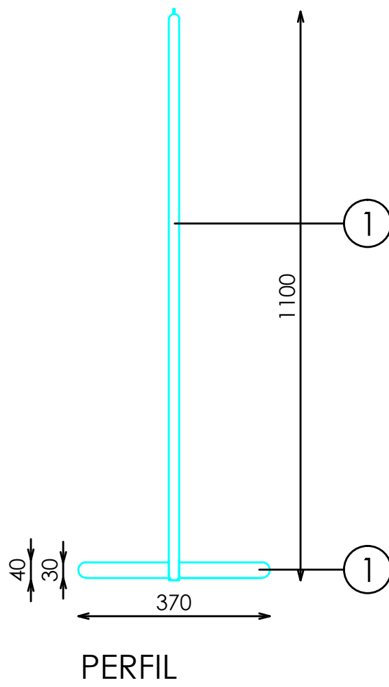
PERFIL
