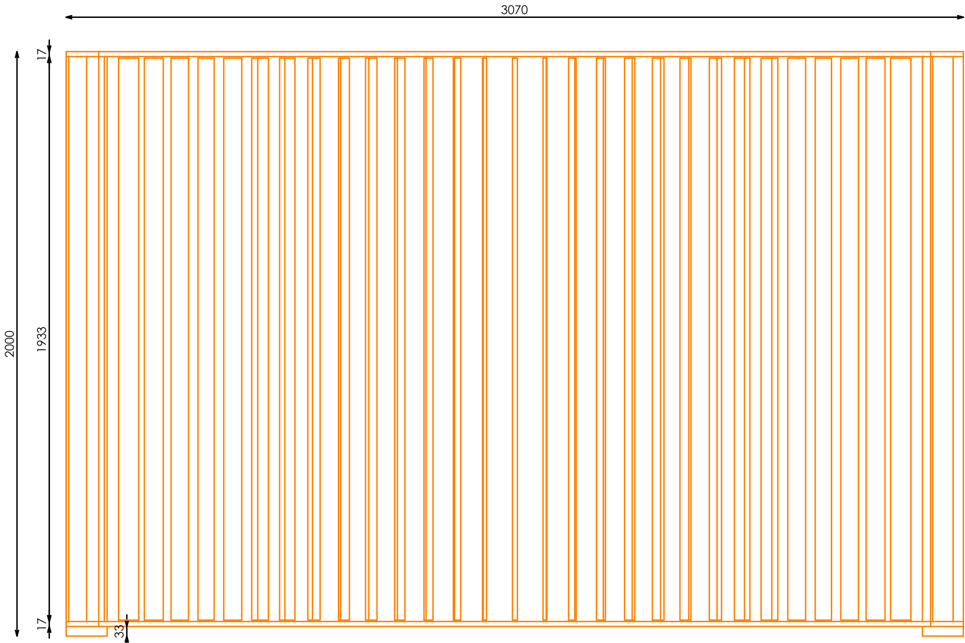
ALZADO
