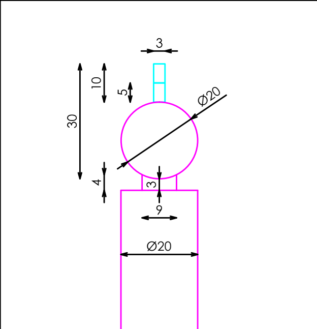
DETALLE B
