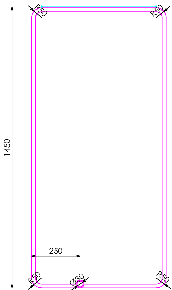
ALZADO
