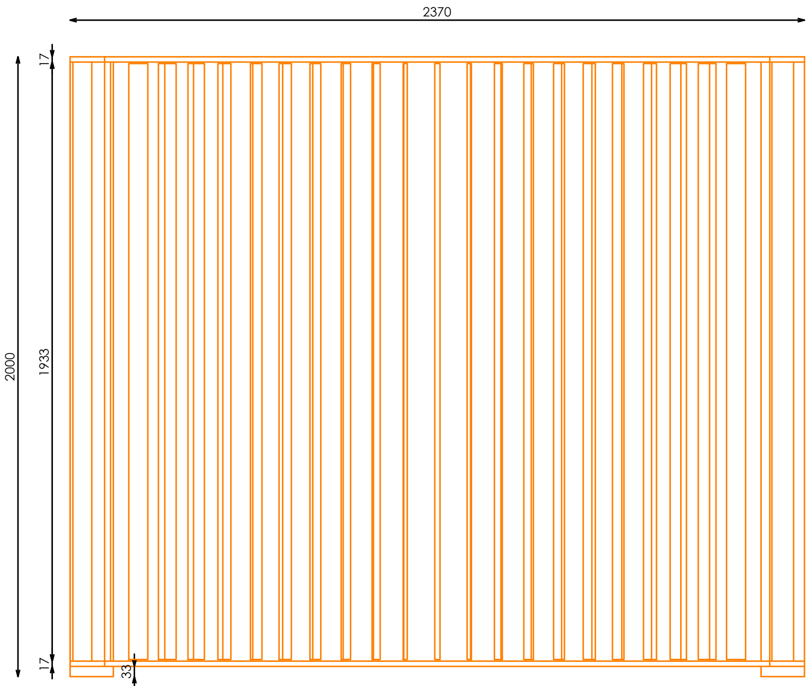
ALZADO
