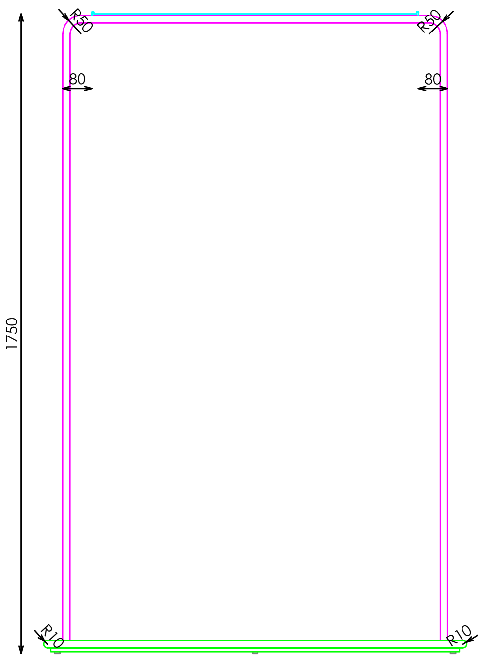
ALZADO
