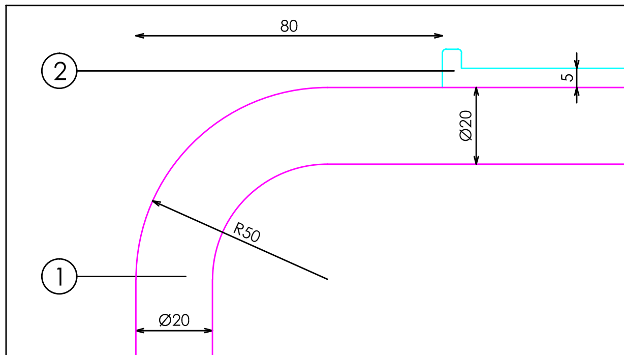
DETALLE A
