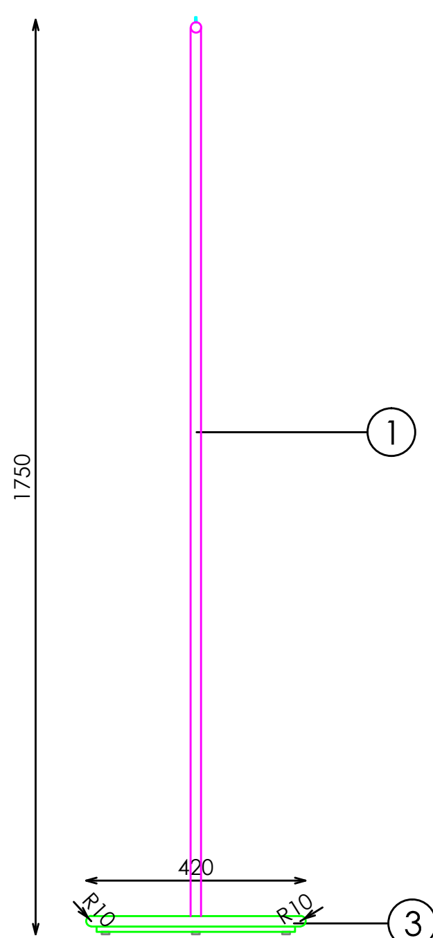
PERFIL
