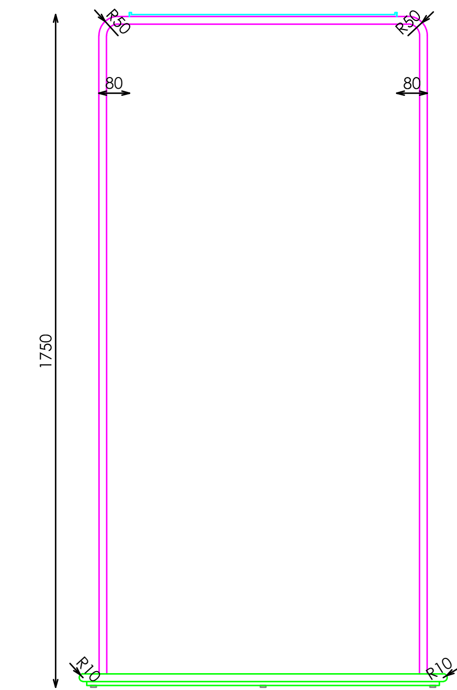
ALZADO
