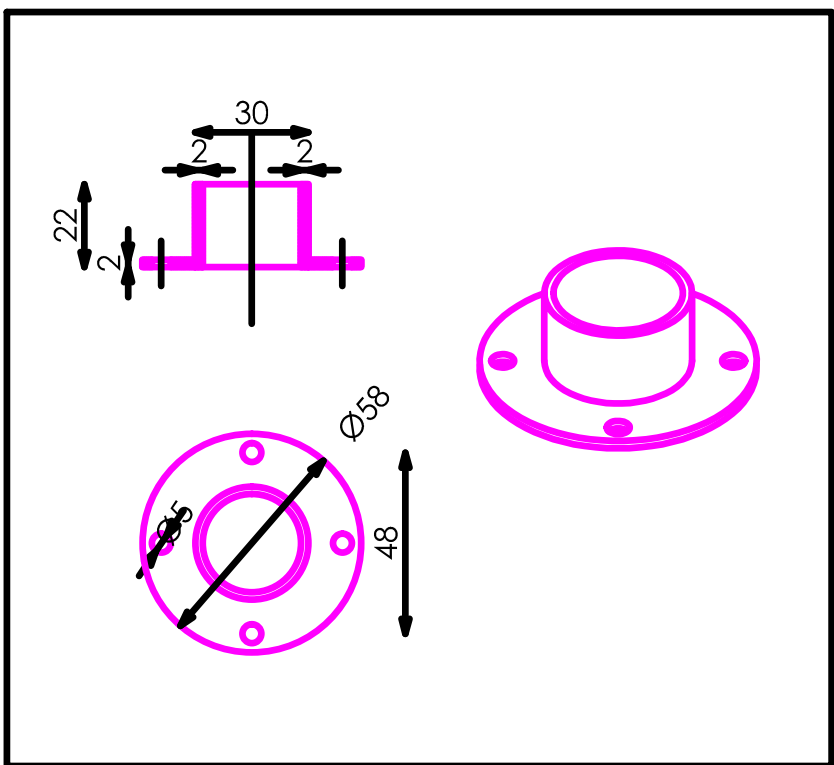
CASQUILLO EMBELLECEDOR
