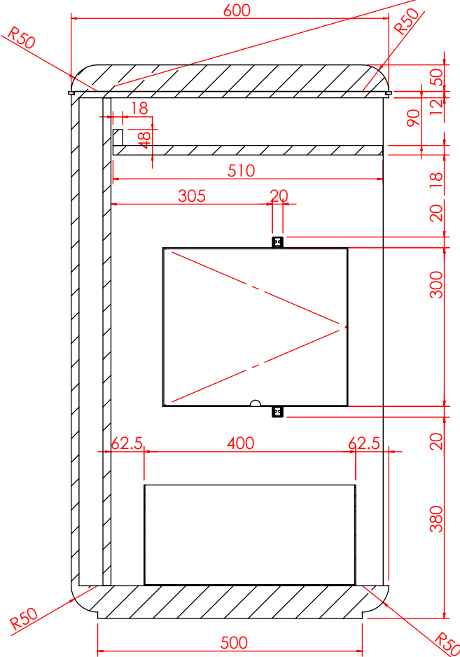
剖面 AG-AG
