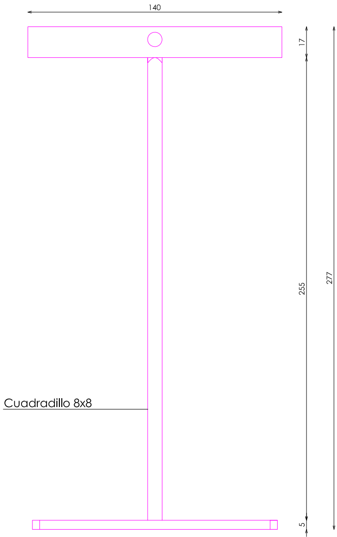
ALZADO
