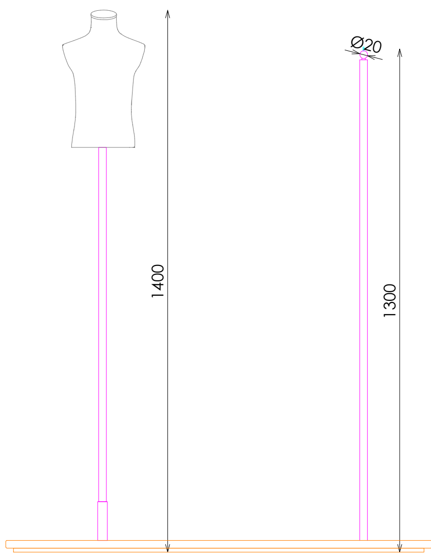
ALZADO
