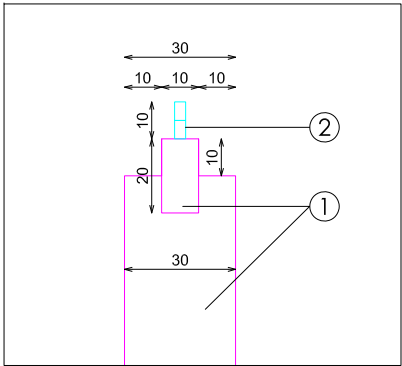
DETALLE A
