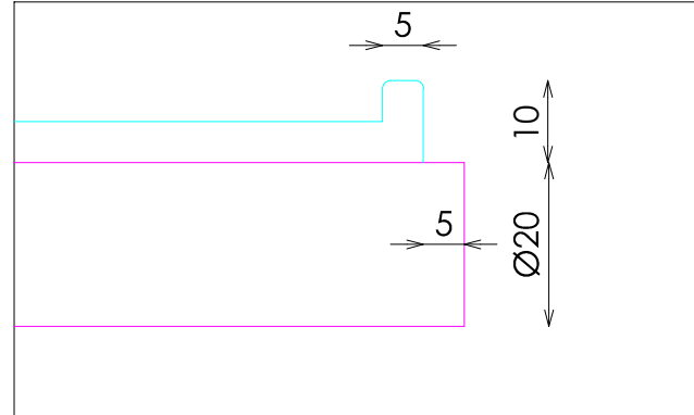
DETALLE ANTIROCE
