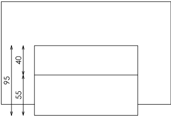
PERFIL DCHO
